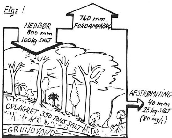
Fig. 1: Vegetationen fordampner næsten al vandet, grundvandsstanden er lav, og der er oplagret store mængder salt i jorden.
