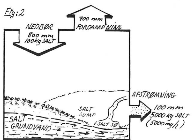
Fig. 2: Den naturlige vegetation er ryddet, fordampningen mindre, grundvandsstanden stiger, og der sker både en udvaskning og opløsning af det opmagasinerede salt.
